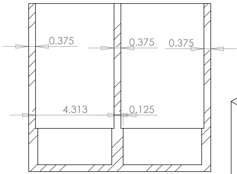
SECTION B-B SCALE 1 : 3
