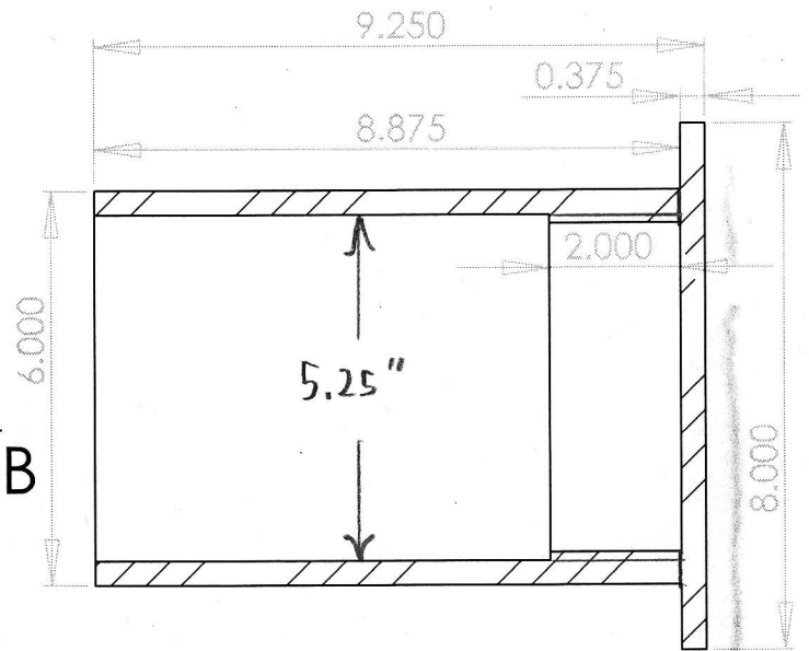
SECTION A-A SCALE 1 : 3
